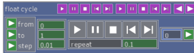
Obrázek 4.9: Komponenta cycle.
