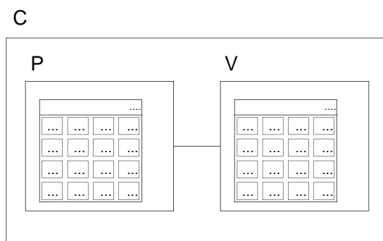
Obrázek 3.7: Transformace kamery
