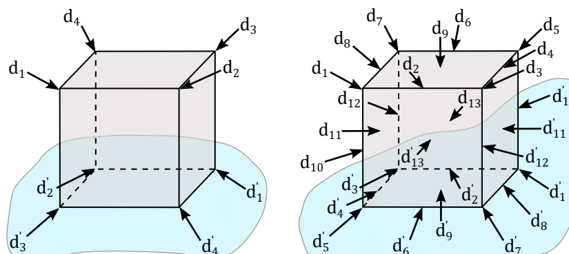
Obrázek 3.2: Ukázka reprezentativních směrů k předpočítání pořadí průchodu synů při traverci BVH. Pro 4 a 13 směrů paprsků společně se směry symetrie při průchodu v opačném pořadí v modrém poli.
