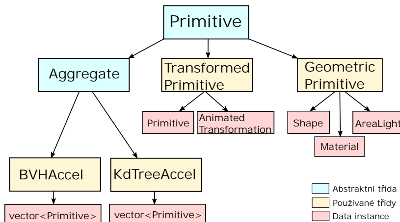
Obrázek 2.3: Hierarchie abstraktní třídy Primitive v PBRT.
