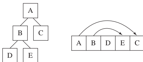
Obrázek 2.4: Ukázka přestavby binární hierarchie ze stromové struktury do lineárního pole (převzato z [PJH16]).
