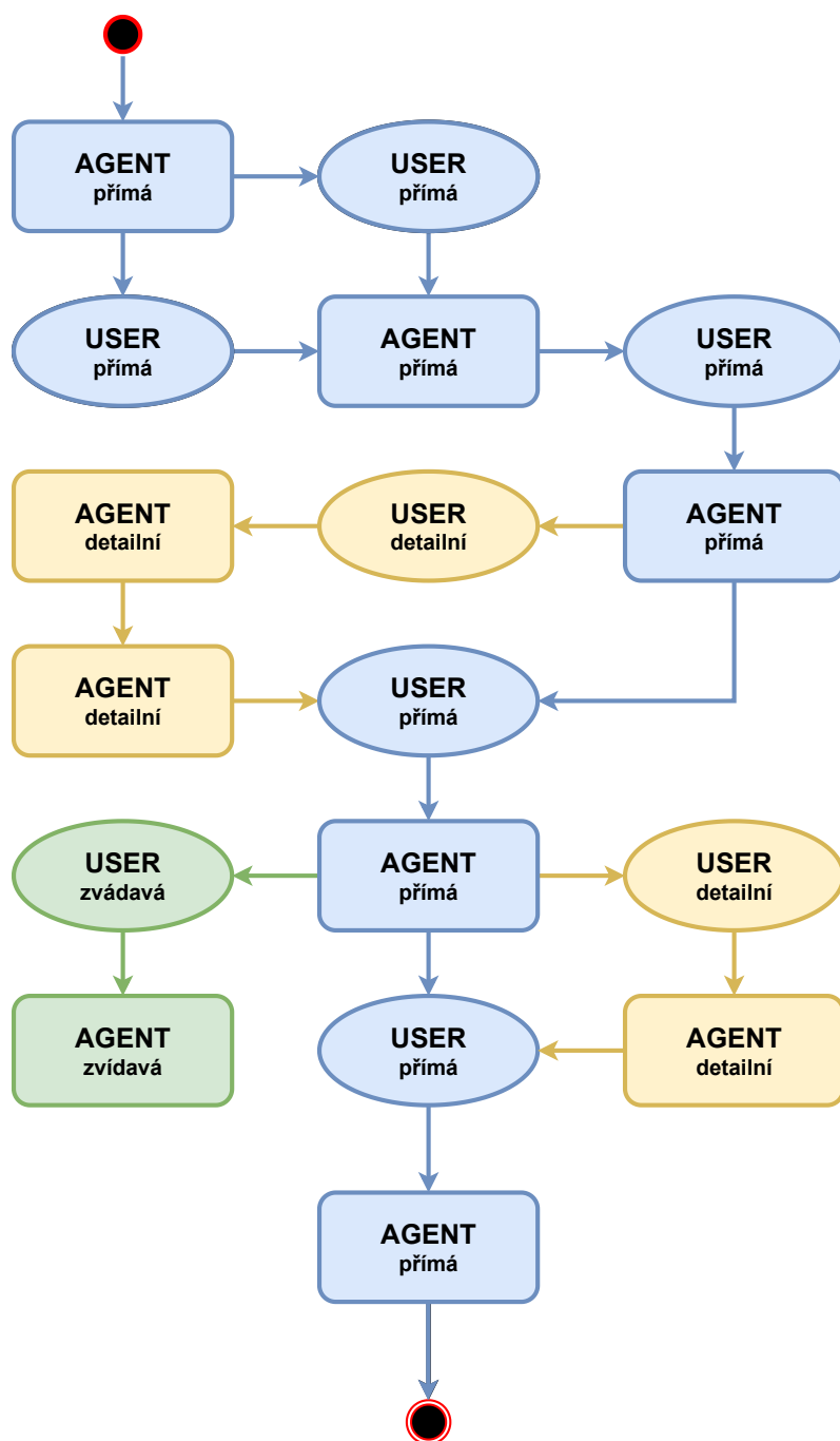
Obrázek C.4: Konverzační diagram zachycující různé cesty
